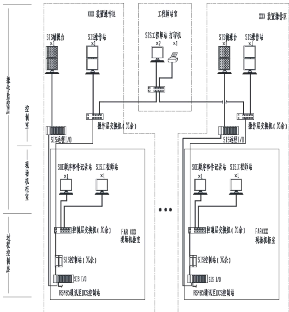
图 3 化工厂安全仪表系统网络典型结构图
