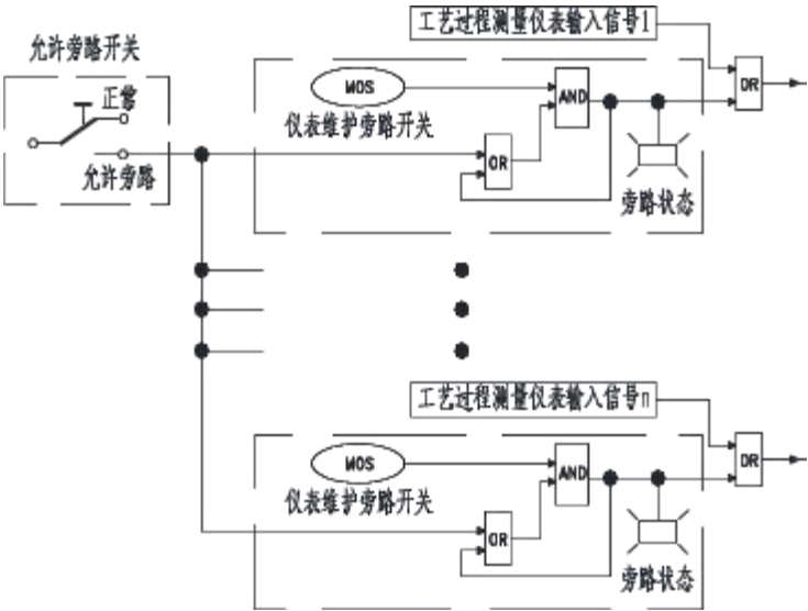
图 10 软件仪表维护旁路开关和硬件允许旁路开关典型设置示例
