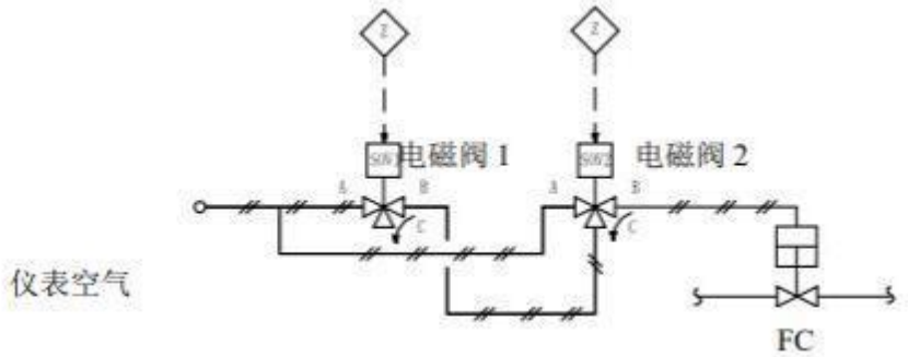
图 9 气动切断阀控制电磁阀可用性冗余结构配置示例
