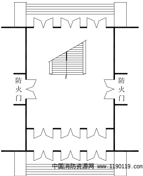
图 5 扩大封闭楼梯间示意图
